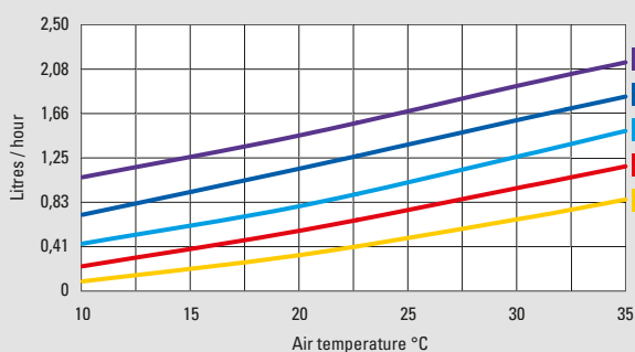
Dehumidification performance DS 30
