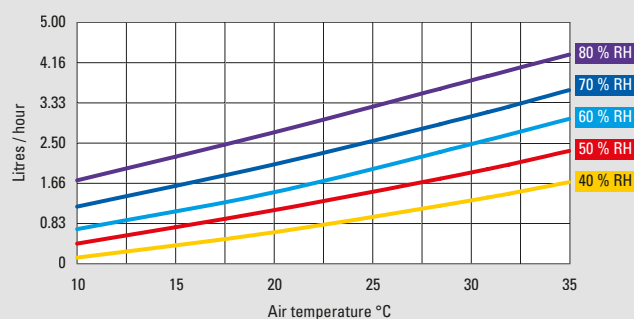
Dehumidification performance DS 60
